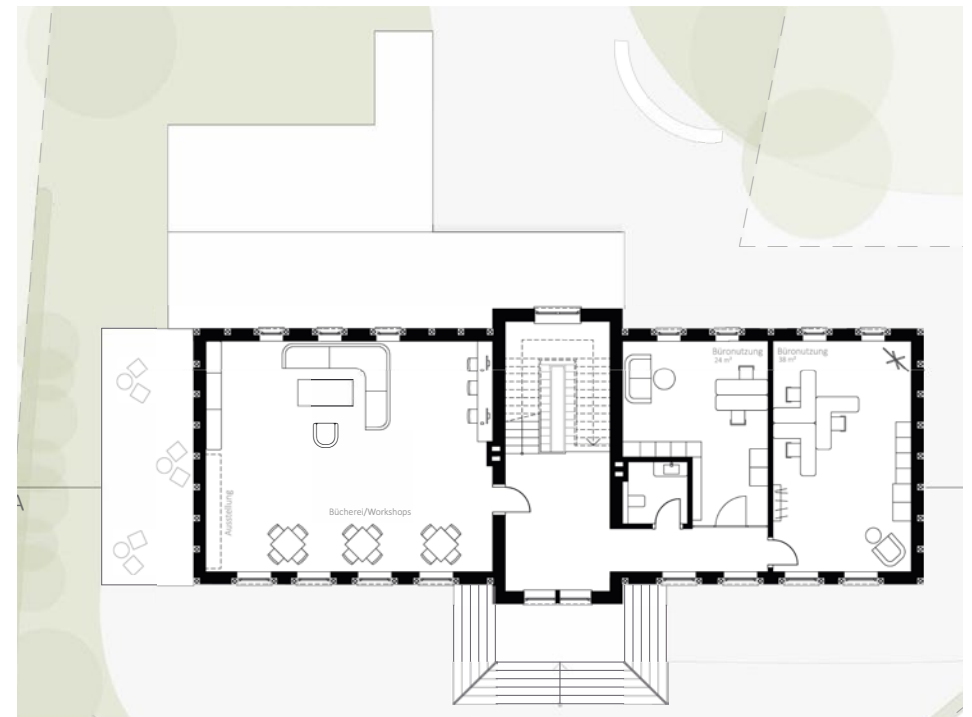
Grundriss 1. OG
