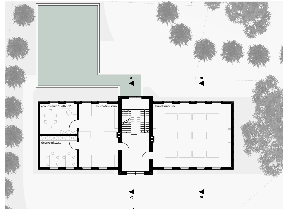
Grundriss 1. OG
