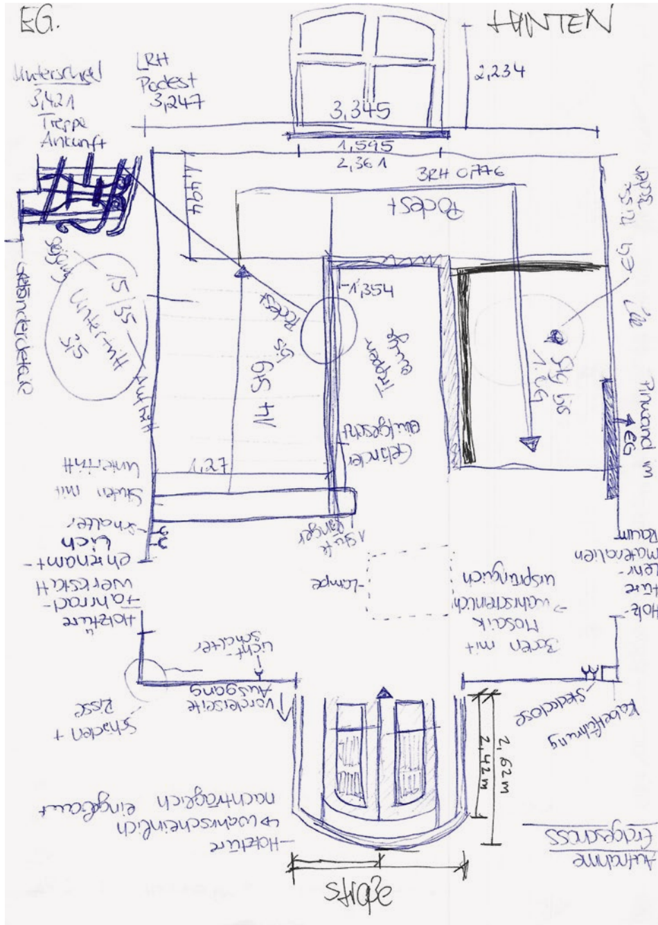
Abb. 33: Skizze des Treppenhauses, Ahmet-Can Canbaz, Jana Steuer, Nina Tenhaken, 2022. Die Zeichnung mit Maßangaben und Vermerk von baulichen Besonderheiten diente als Arbeitshilfe für das Aufmaß der Grundrisse und das Raumbuch.
