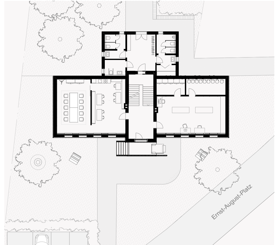
Grundriss EG
