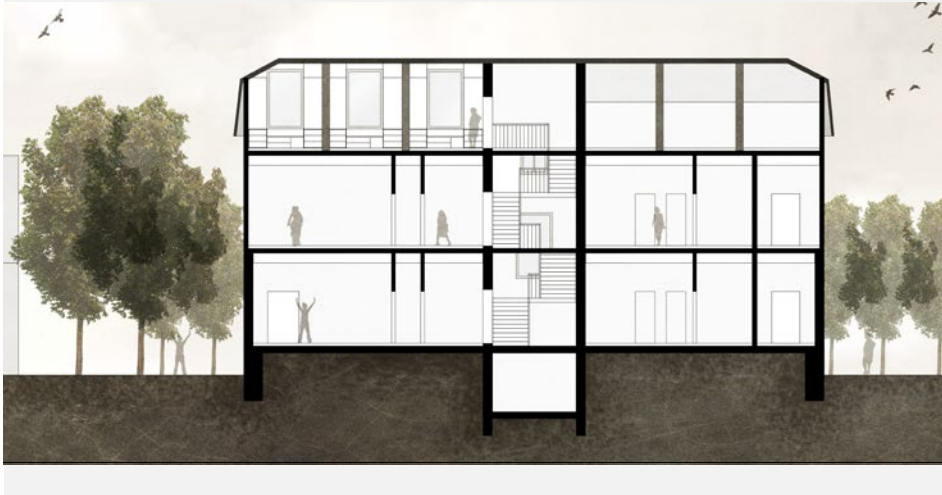
Schnitt
