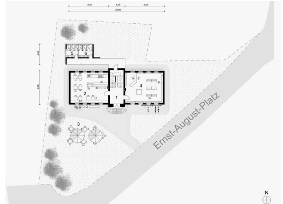
Grundriss EG
