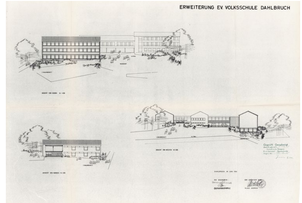
Abb. 37: Zweiter Bauabschnitt des Schulneubaus an der Hochstraße, Plan, Klaus Andrick, Juni 1964
