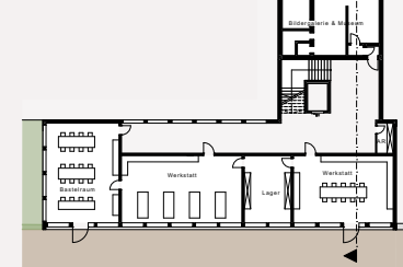
GRUNDRISS UNTERGESCHOSS
