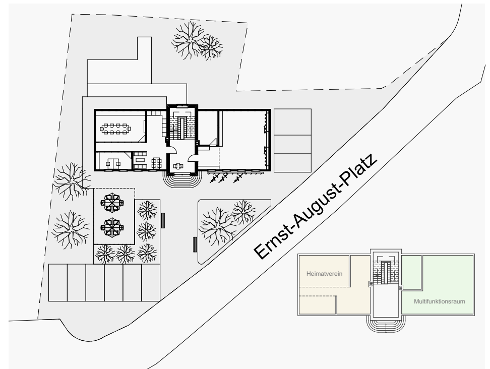
Grundriss 1. OG
