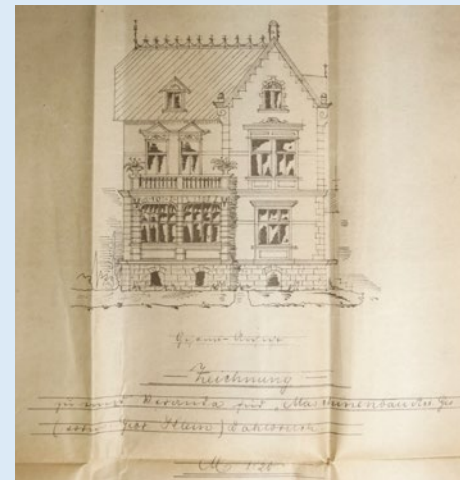
Abb. 28: Aufriss eines Wohnhauses in Dahlbruch, Anbau einer Veranda von Hermann Giesler sen., Ausschnitt Entwurfszeichnung, 11.5.1905
