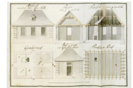
Abb. 5: Plan eines steinernen Schulhauses, nicht ausgeführt, Februar 1784
