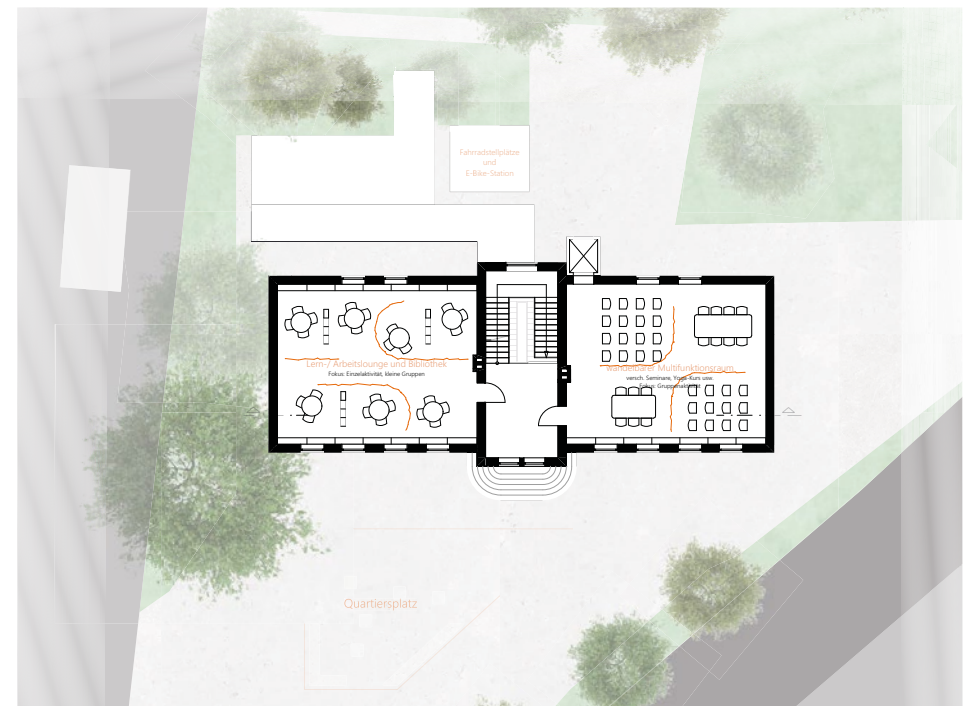
Grundriss 1. OG
