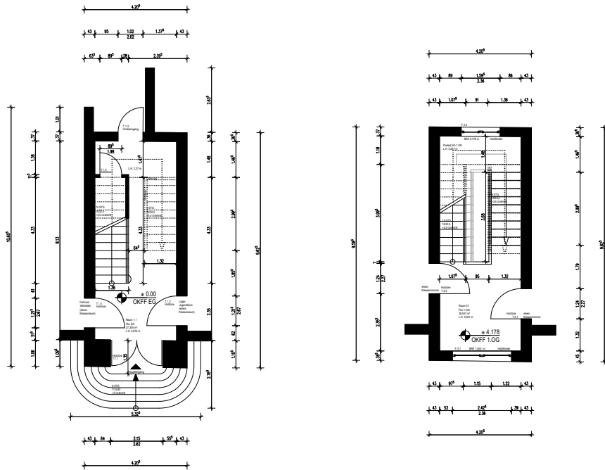
Abb. 30: Grundriss EG und 1. OG des Treppenhauses der Alten Schule, Ahmet-Can Canbaz, Jana Steuer, Nina Tenhaken, 2022. Die Zeichnung wurde auf Grundlage des Handaufmaßes mit einem CAD-Programm von den Studierenden erstellt.
