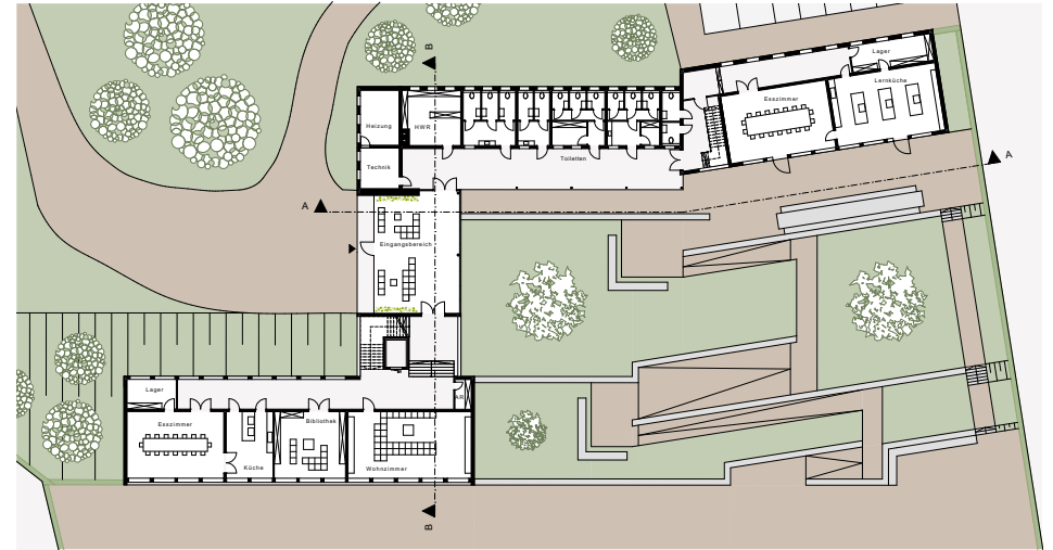
GRUNDRISS UNTERGESCHOSS
