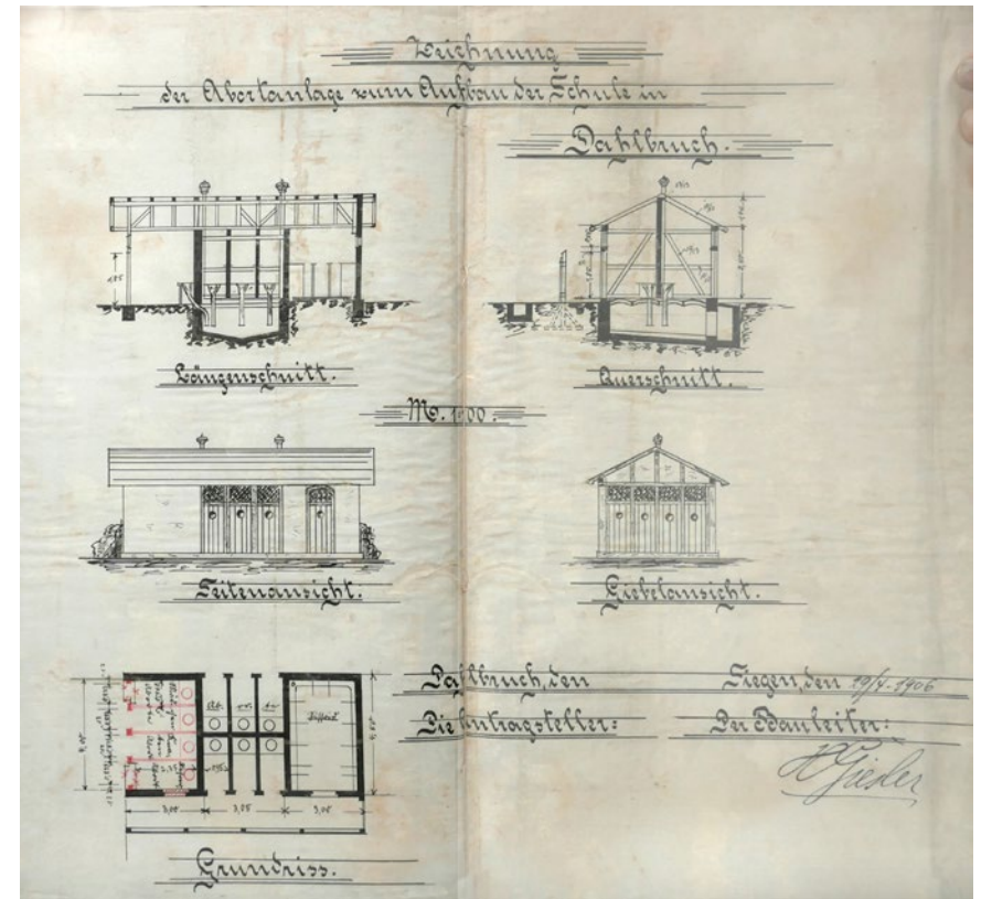
Abb. 22: Toilettenhäuschen, Eintragung zum Umbau durch Hermann Giesler sen., 29.4.1906, auf Grundlage eines Plans von 1897
