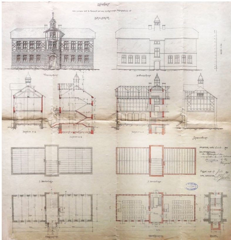
Abb. 21: Schulhausaufstockung, Plan, Hermann Giesler sen., 19.7.1905
