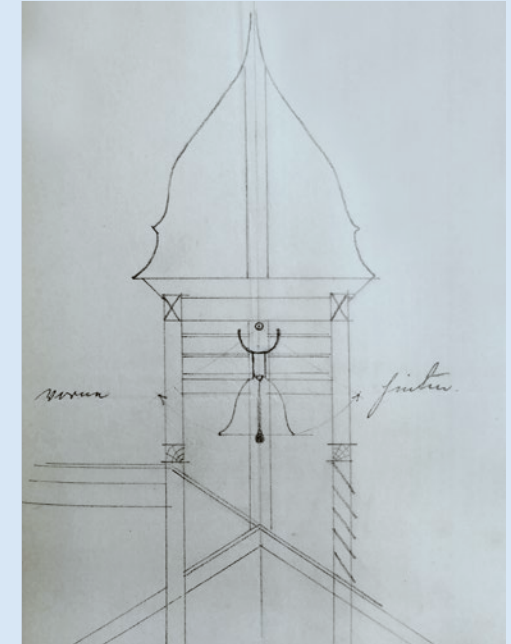
Abb. 16: Dachreiter mit Schulglocke, Ausschnitt Skizze, Hermann Giesler sen., Februar 1907
