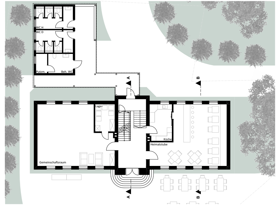
Grundriss EG
