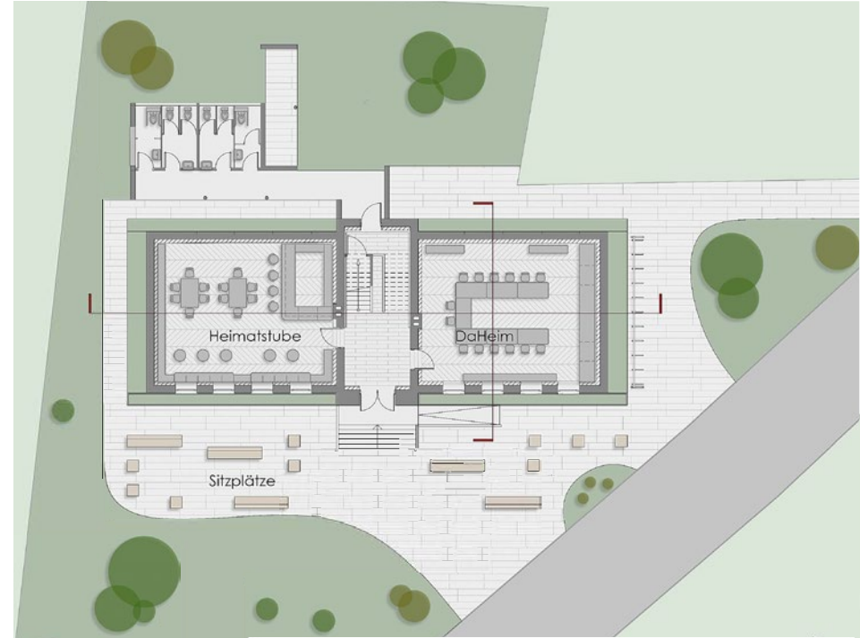
Grundriss EG
