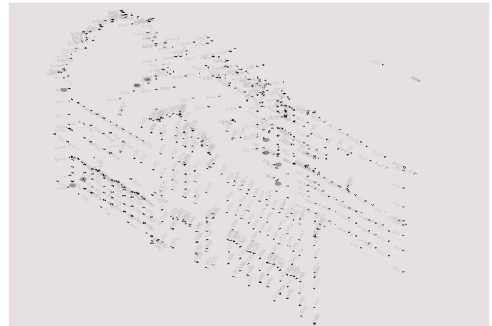
Abb. 32: Punktwolke des Schulhauses, Screenshot 2023. Die mit dem Tachymeter aufgenommenen Messpunkte an der Fassade des Gebäudes wurden in das CAD-Programm übertragen. Um das gesamte Gebäude zu erfassen, wurde das Tachymeter mehrfach versetzt und für jeden Standort eine separate Datei angelegt. Zudem mussten Referenzpunkte festgelegt werden, die von unterschiedlichen Standpunkten aufgenommen wurden. Sie halfen, die einzelnen Dateien im CAD-Programm zu einer Punktwolke des gesamten Gebäudes zusammenzusetzen.
