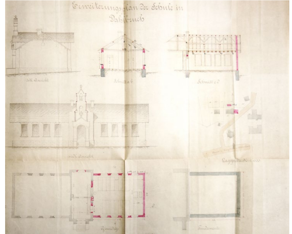
Abb. 14: Schulhaus mit dem ergänzten Klassenraum (rot markiert), Entwurfszeichnung, J. Kolb, Februar 1897
